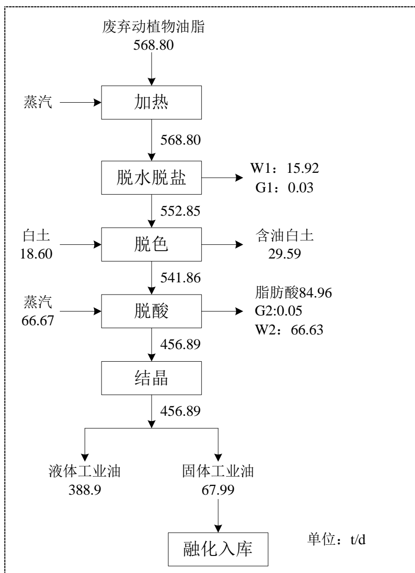
图 3.5-3 废弃动植物油脂前处理物料平衡图
