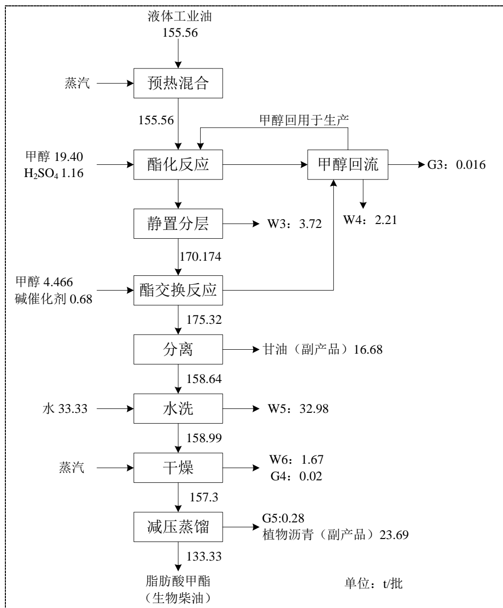
图 3.5-4 脂肪酸甲酯（生物柴油）物料平衡图
