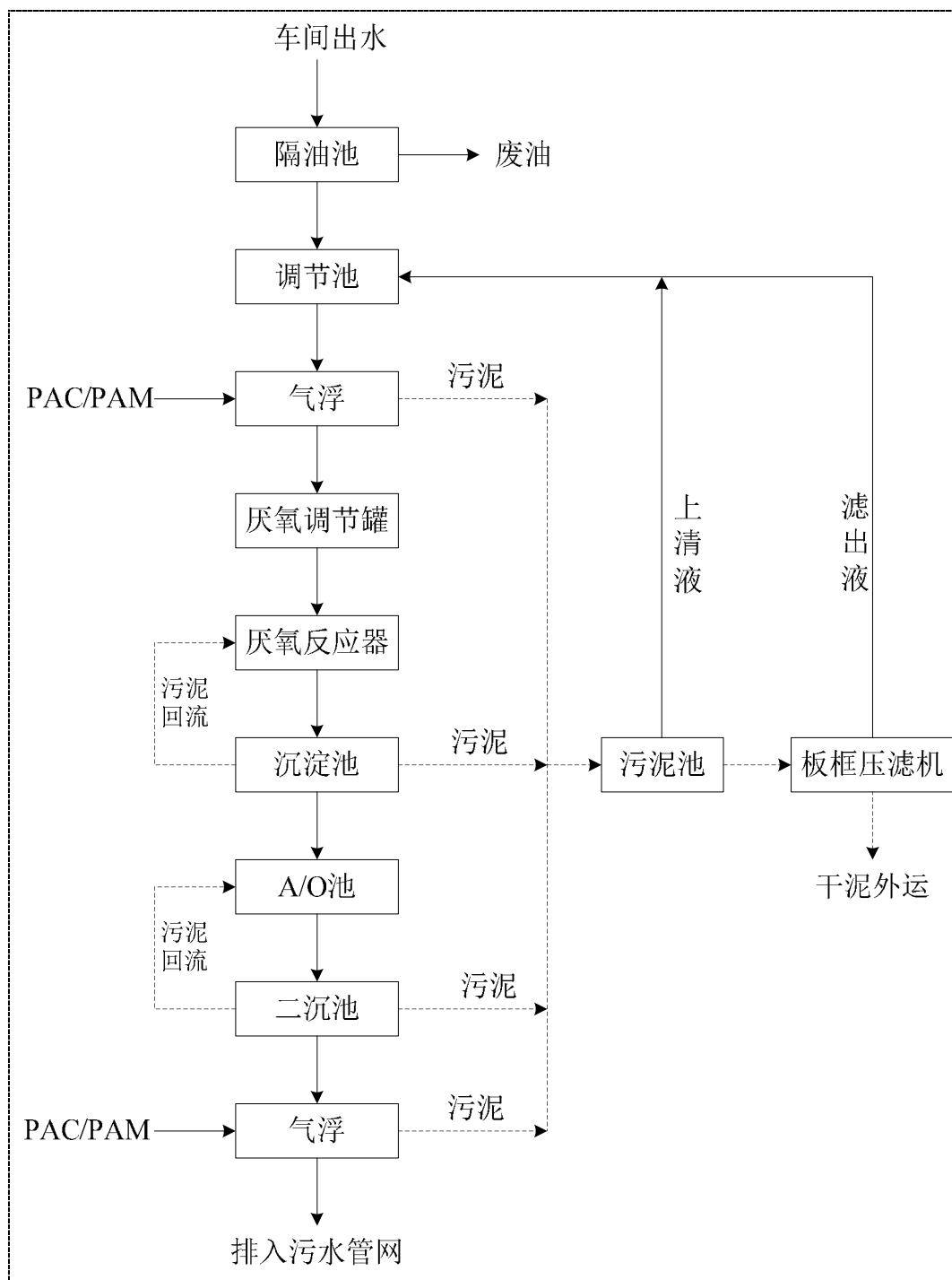
图 6.2-1 废水处理工艺流程图
