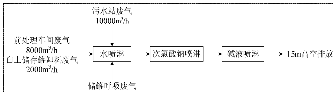
图 6.2-4 储罐废气、污水站恶臭废气处理流程图
