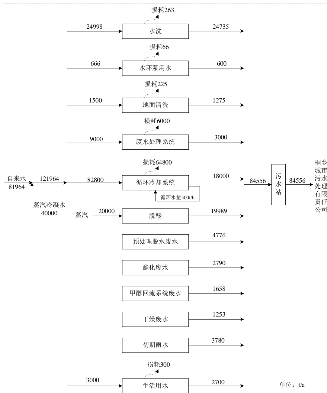
图 5.5-19 本项目水平衡图
