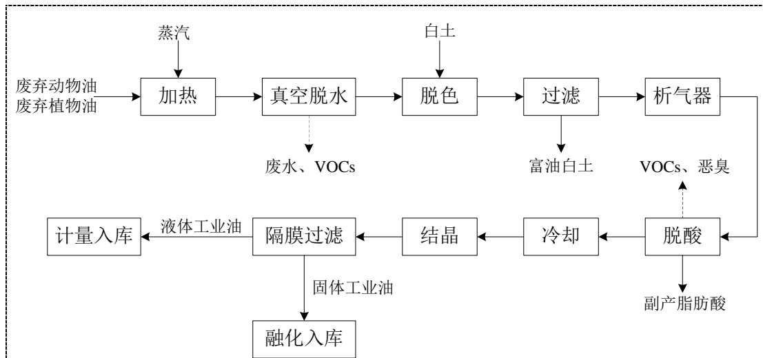
图 3.5-1 废弃动植物油脂前处理生产工艺流程图
